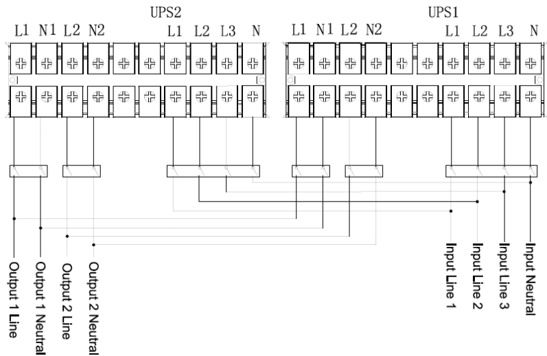
Abbildung 16: Anschlussplan für Parallelbetrieb von zwei XANTO 20000 3/1
