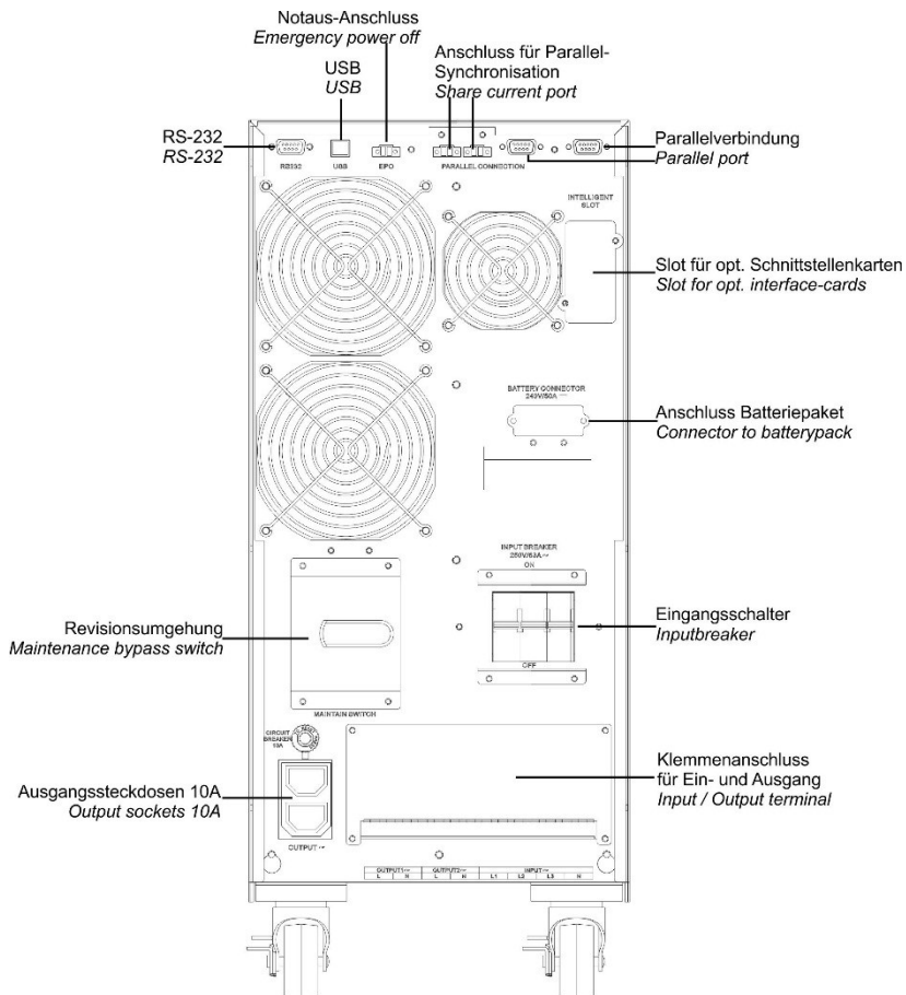
Abbildung 29: Rückansicht XANTO 10000 3/1
