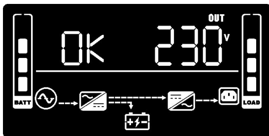
Abbildung 19: Display Normalbetrieb
