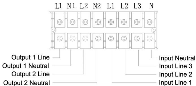
Abbildung 12: Klemmleiste XANTO 10000 3/1
