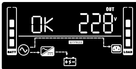
Abbildung 23: Display Bypassbetrieb
