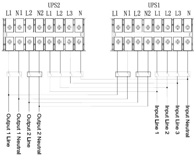
Abbildung 15: Anschlussplan für Parallelbetrieb von zwei XANTO 10000 3/1
