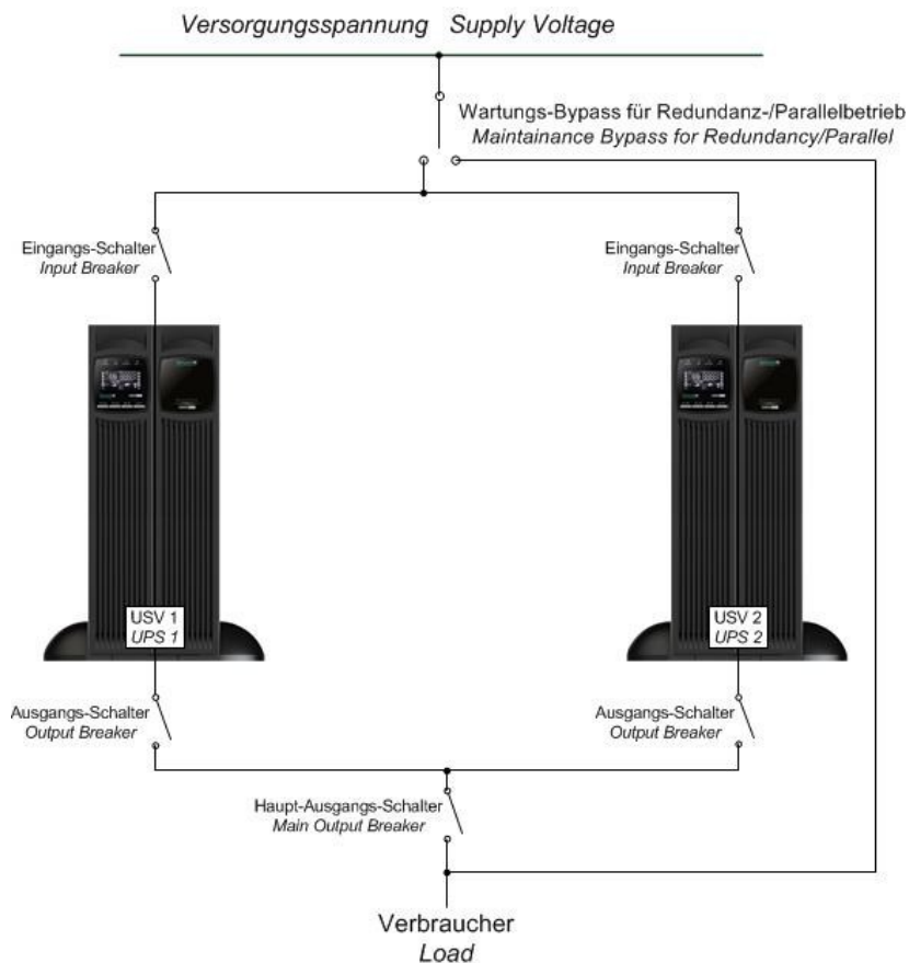
Abbildung 17: Blockschaltbild Parallelschaltung
