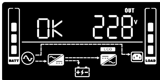
Abbildung 22: Display Hocheffizienzbetrieb
