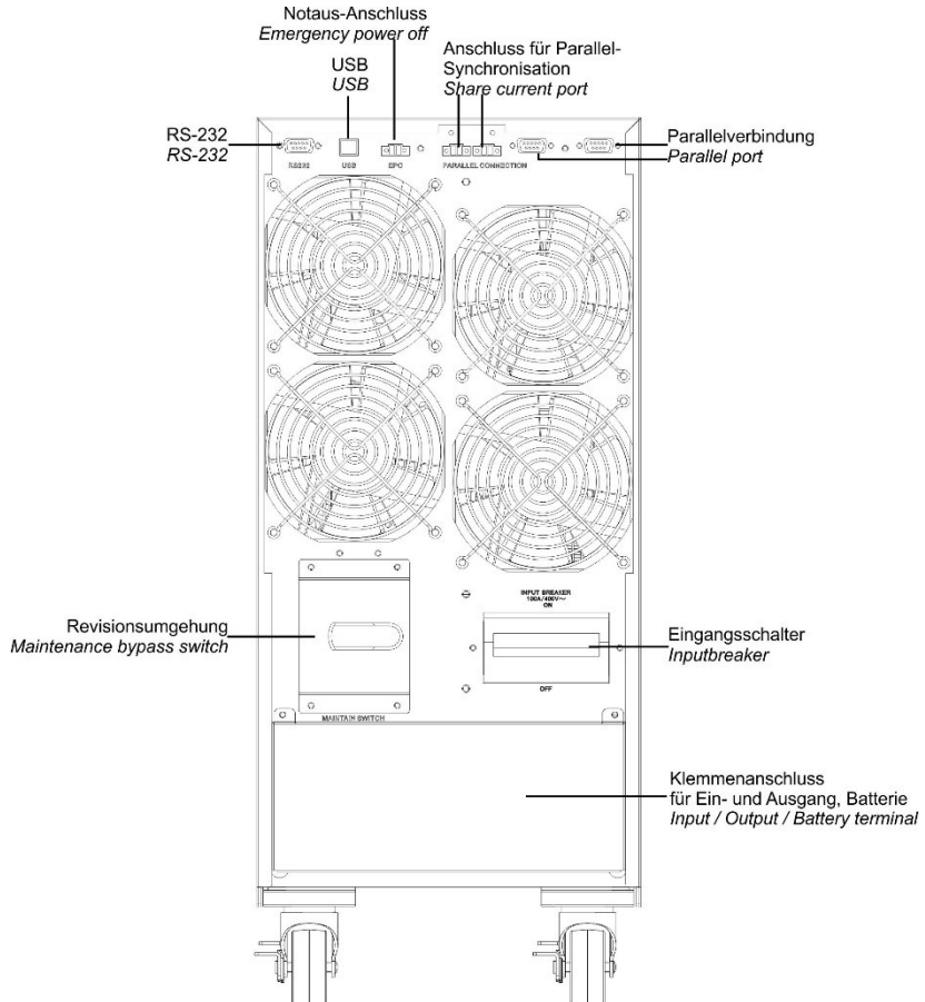
Abbildung 30: Rückansicht XANTO 20000 3/1
