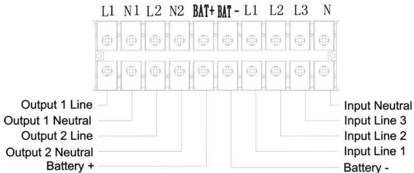
Abbildung 13: Klemmleiste XANTO 20000 3/1
